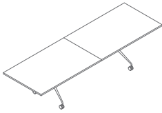
PCP05 3200 / 1000 / 740** 101 kg
