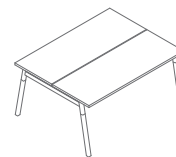
BOW56 1600 / 1210 / 740 58 kg
