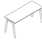
BOW16 1600 / 600 / 740 31.5 kg
